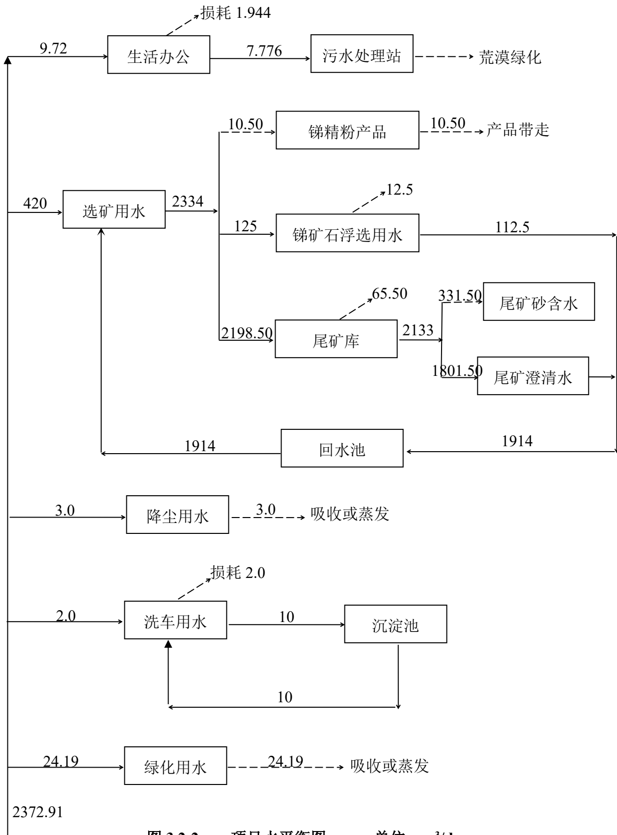
图 3.2-2 项目水平衡图 单位: m³/d
